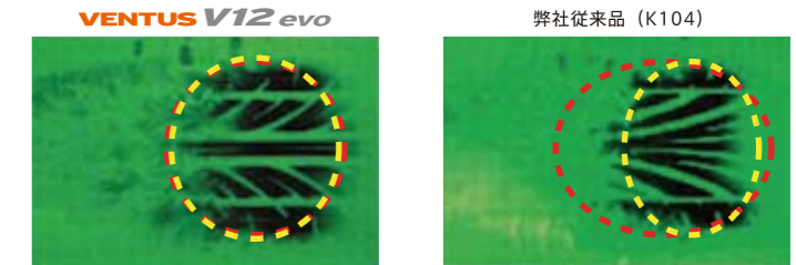
【実車ハイドロプレーニングテスト (速度: 100km/h・水深: 10mm)】
